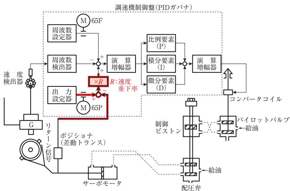
図2 ガバナの動作説明図
