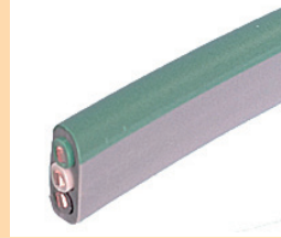
▲ No.14 600V ビニル絶縁ビニルシース ケーブル 平形 2.0mm 3心 (黒・白・緑)
