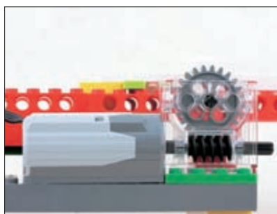
写真8 モーターとウォームギア
