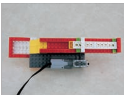
写真7 上から見た様子
